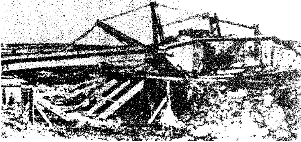
جسر انقراض بريطاني في الحرب العالمية الأولى (دبابة مارك - هـ)
