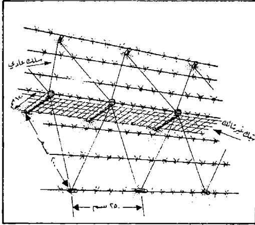
سياج شائك مع شبك غير شائك
