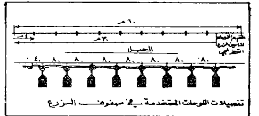
حبل لزرع حقل ألغام نظامي
