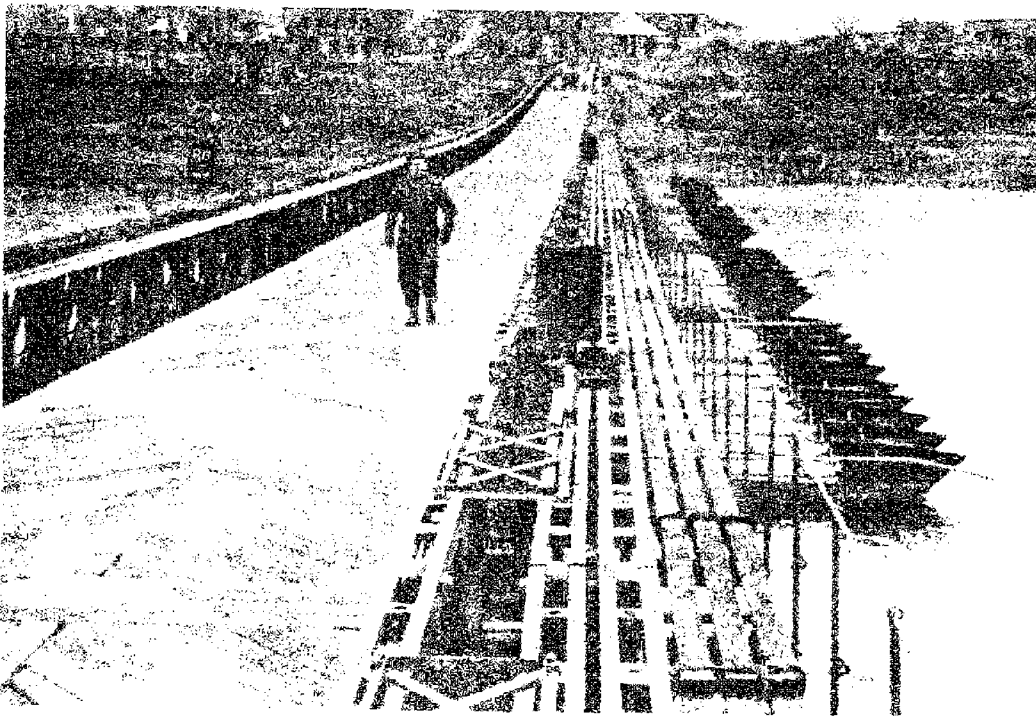
جسر « بيللي » عائم حمولة ٨٠ طناً
