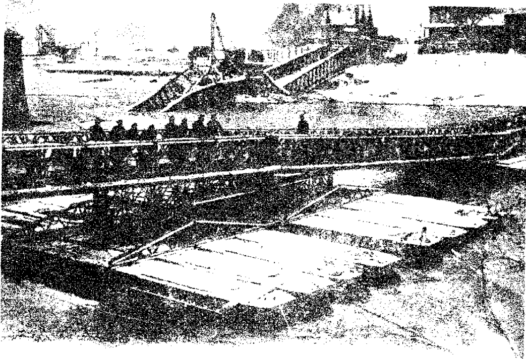
جسر « بيللي » على دعائم عائمة
