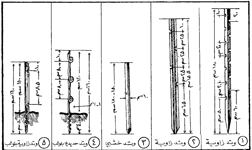
أوتاد الأسلاك الشائكة
