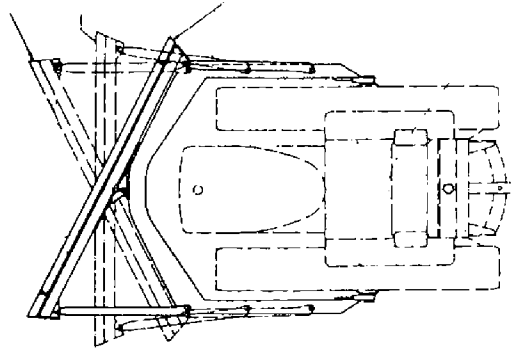
تحويل البلدوزر إلى أنقل دوزر
