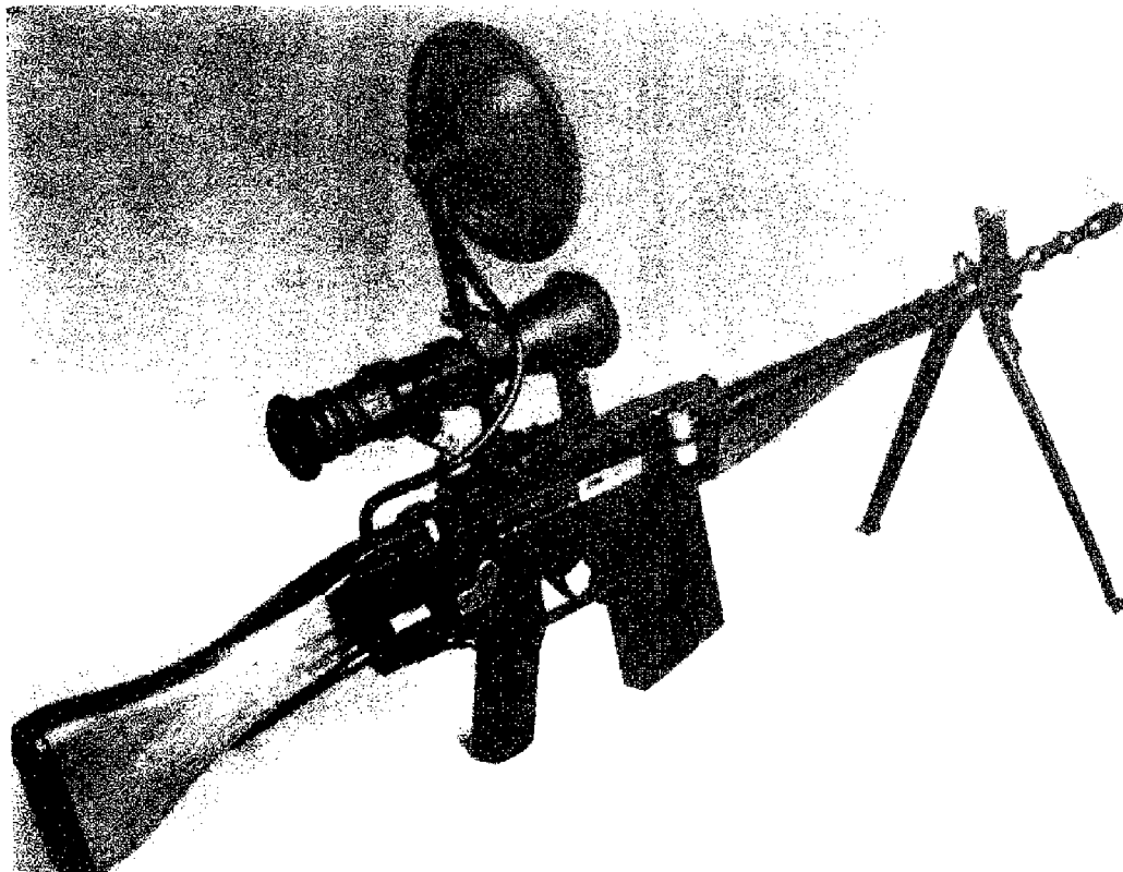
جهاز رؤية ليلية بالأشعة تحت الحمراء مركب على رشاش خفيف
