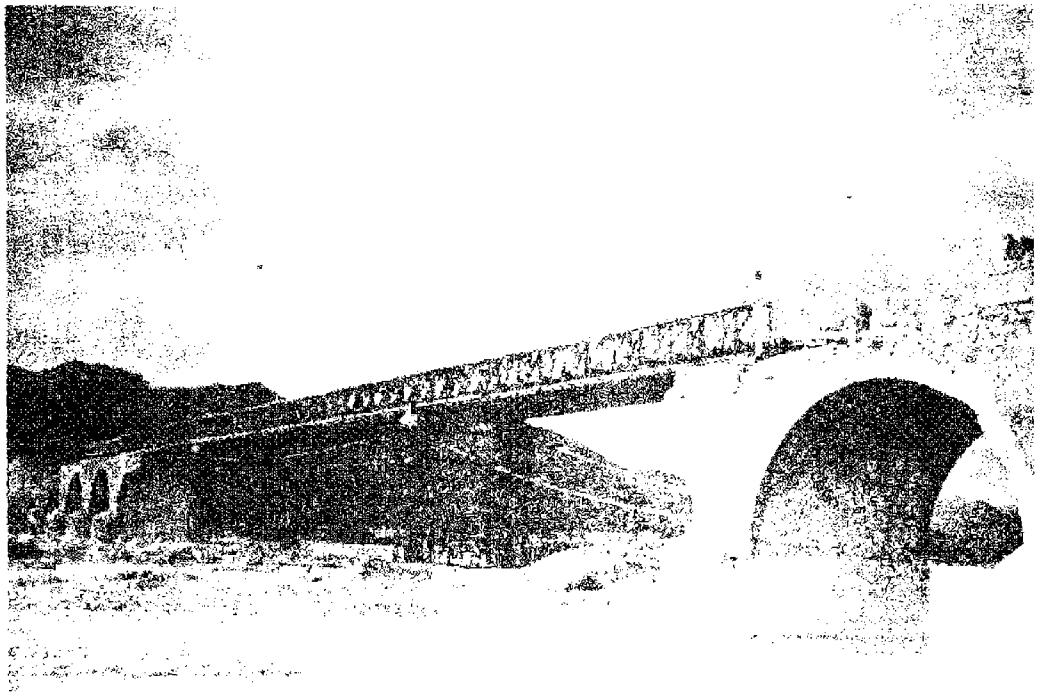
جسر « بيللي » ثابت على نهر فولتورنو
