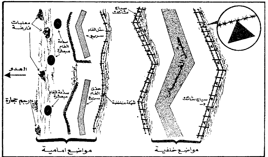
مخطط تحديد وتعليم حقول الألغام من الأمام إلى الخلف
