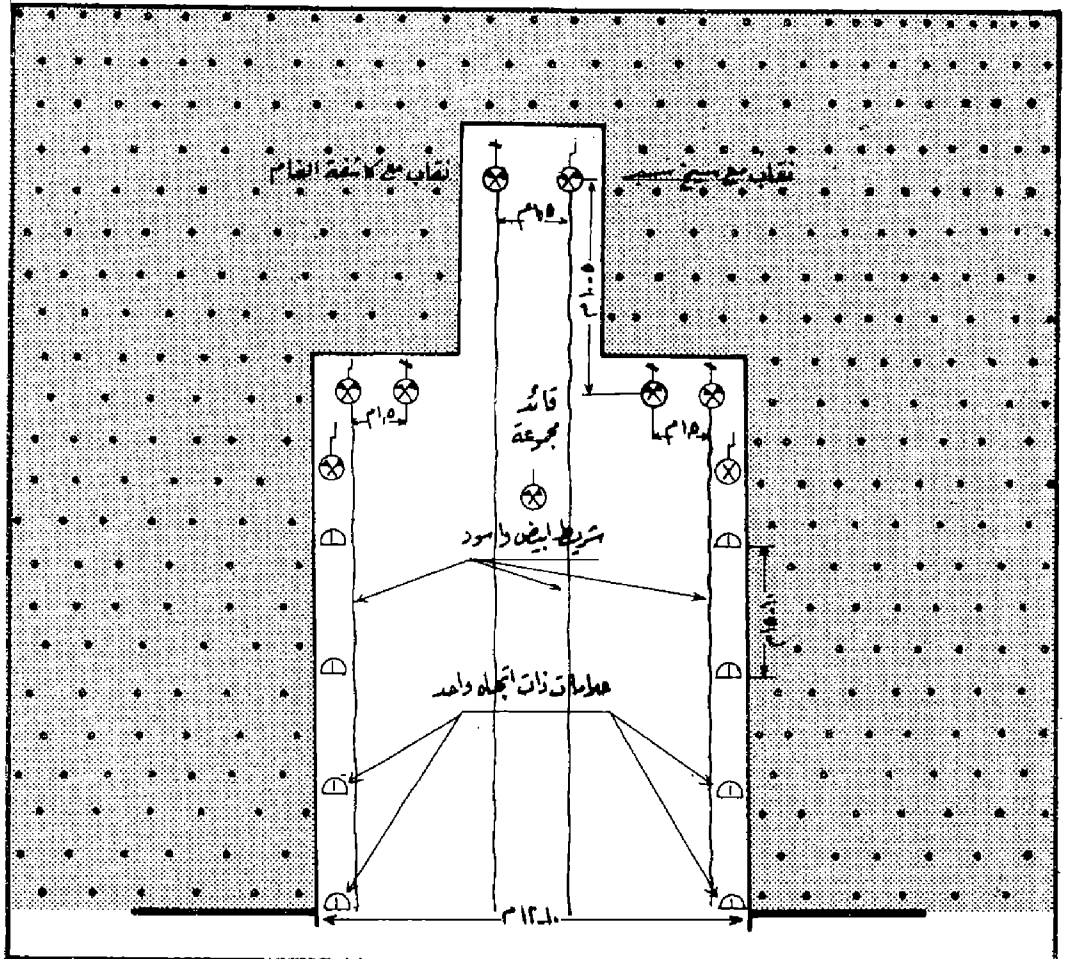
فتح الثغرة في حقل الالغام بالطريقة اليدوية
