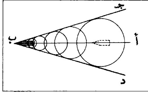
مخروط الماك (الماخ)
